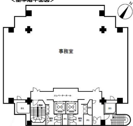
基準階 4～8階
